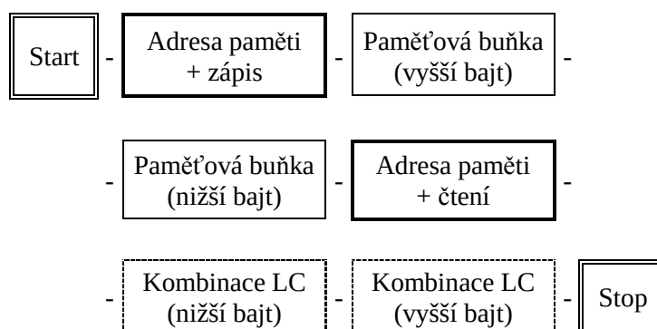
Obr. 4.2: Znáznornění komunikace I 2 C při čtení z paměti EEPROM
